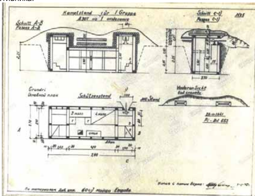
Чертёж немецкого ДЗОТа на одно отделение (из материалов 60-й сд)
